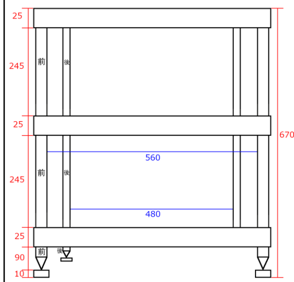
3 段セットの寸法図
